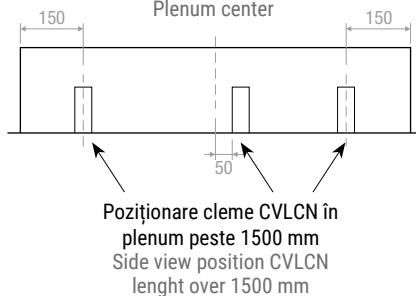
Centrul cutiei plenum Plenum center
