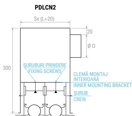
Fixare în plenum cu cleme de prindere CVLCN Fixing the plenum by inner mounting brackets CVLCN
