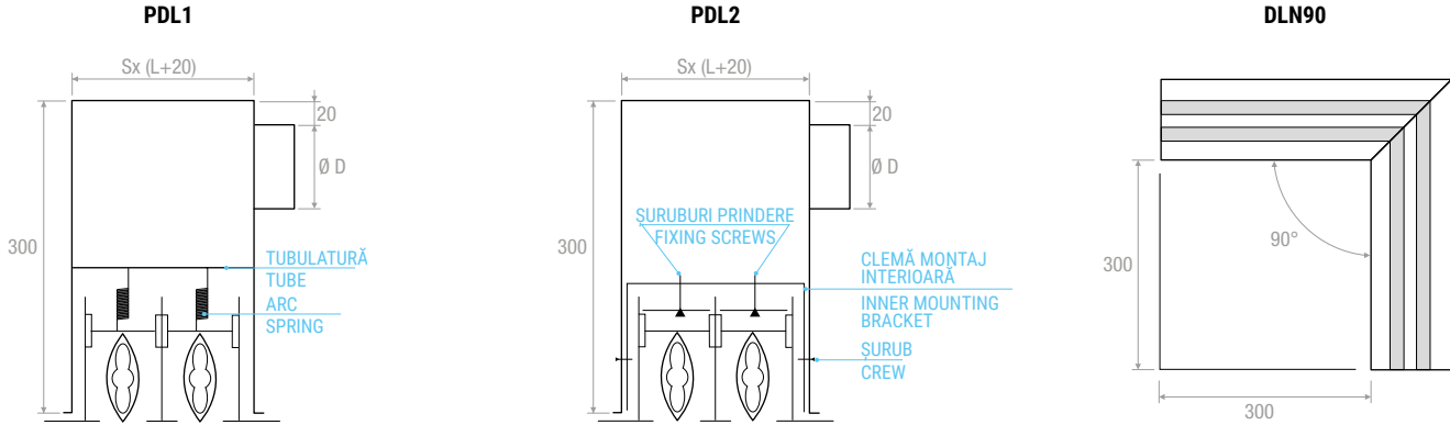
Fixare în plenum cu cleme de prindere CVL Fixing to the plenum by inner mounting brackets CVL
