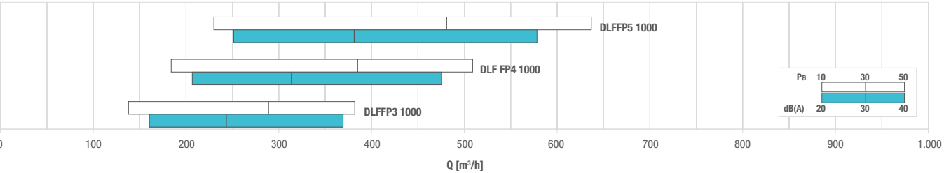
DIAGRAMĂ SELECȚIE RAPIDĂ - QUICK SELECTION DIAGRAM
