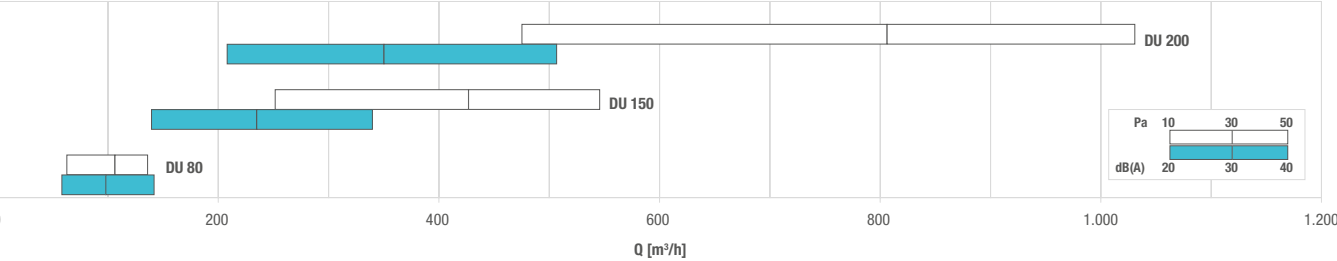
DIAGRAMĂ SELECȚIE RAPIDĂ - QUICK SELECTION DIAGRAM
