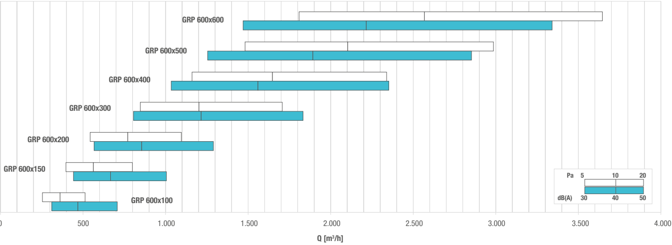
DIAGRAMĂ SELECȚIE RAPIDĂ - QUICK SELECTION DIAGRAM
