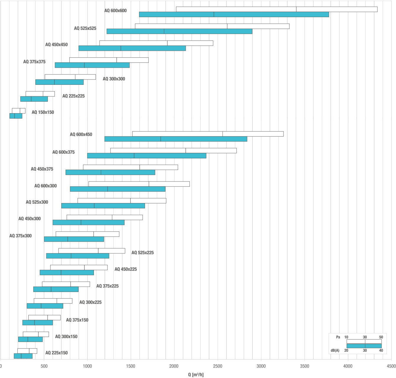
DIAGRAMĂ SELECȚIE RAPIDĂ - QUICK SELECTION DIAGRAM
