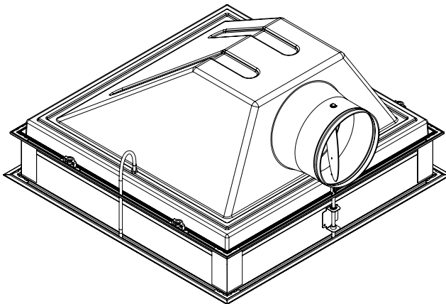
Vedere izometrică - Isometric view
