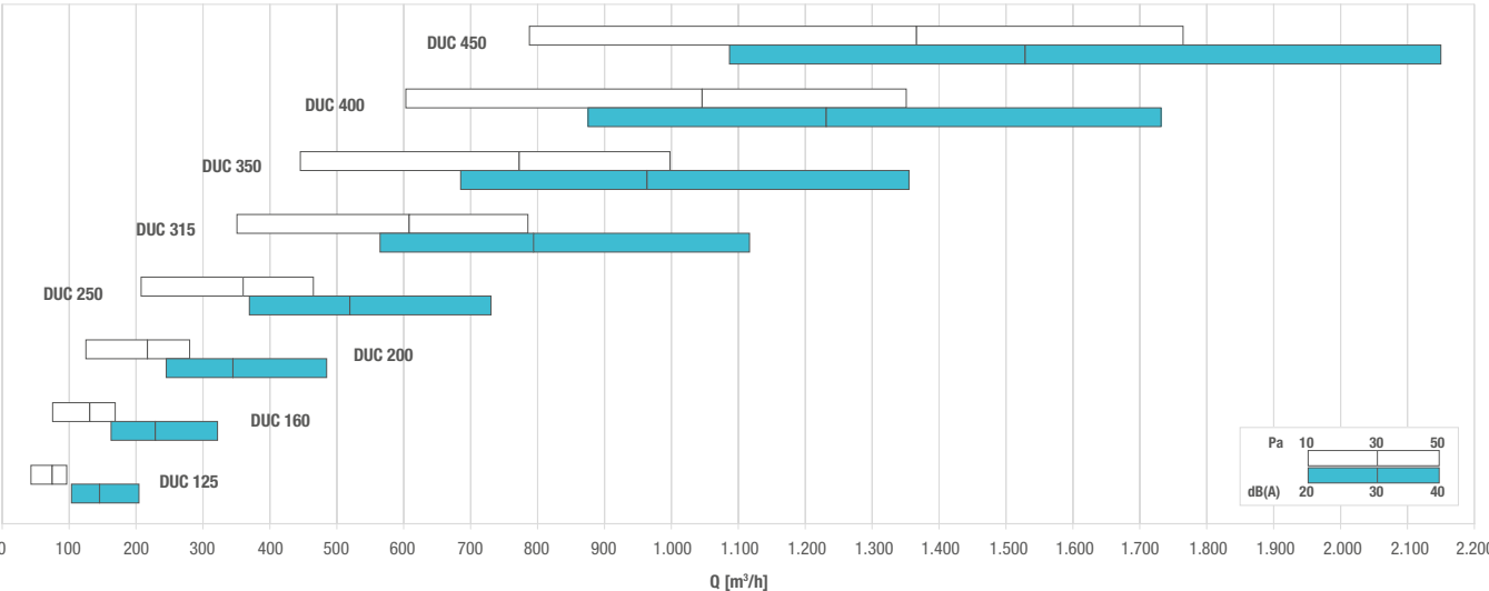
DIAGRAMĂ SELECȚIE RAPIDĂ - QUICK SELECTION DIAGRAM
