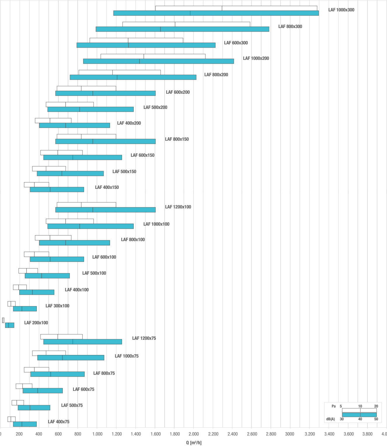
DIAGRAMĂ SELECȚIE RAPIDĂ - QUICK SELECTION DIAGRAM
