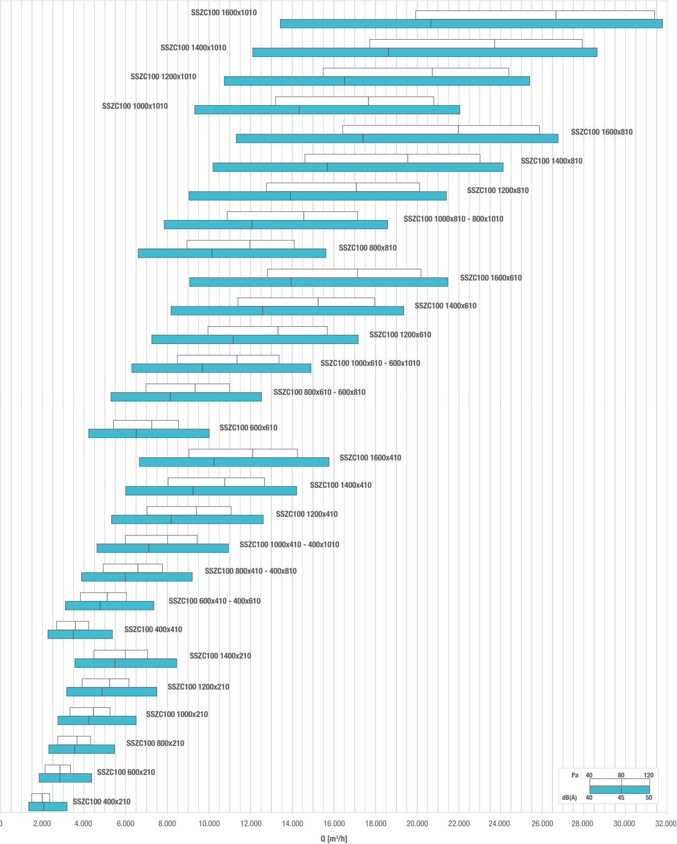
DIAGRAMĂ SELECȚIE RAPIDĂ - QUICK SELECTION DIAGRAM
