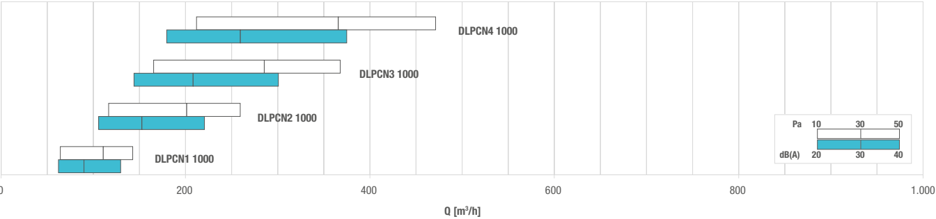
DIAGRAMĂ SELECȚIE RAPIDĂ - QUICK SELECTION DIAGRAM
