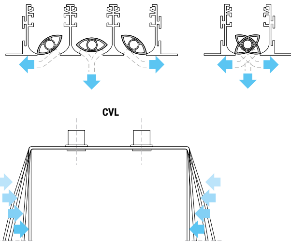
Schimbare configurație CVL în PDL 3 în PDL 2 prin apăsare cu degetul Configuration change CVL to PDL 3 to PDL 2 with finger pressure
