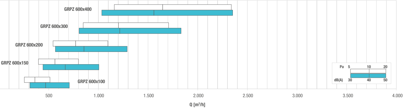
DIAGRAMĂ SELECȚIE RAPIDĂ - QUICK SELECTION DIAGRAM
