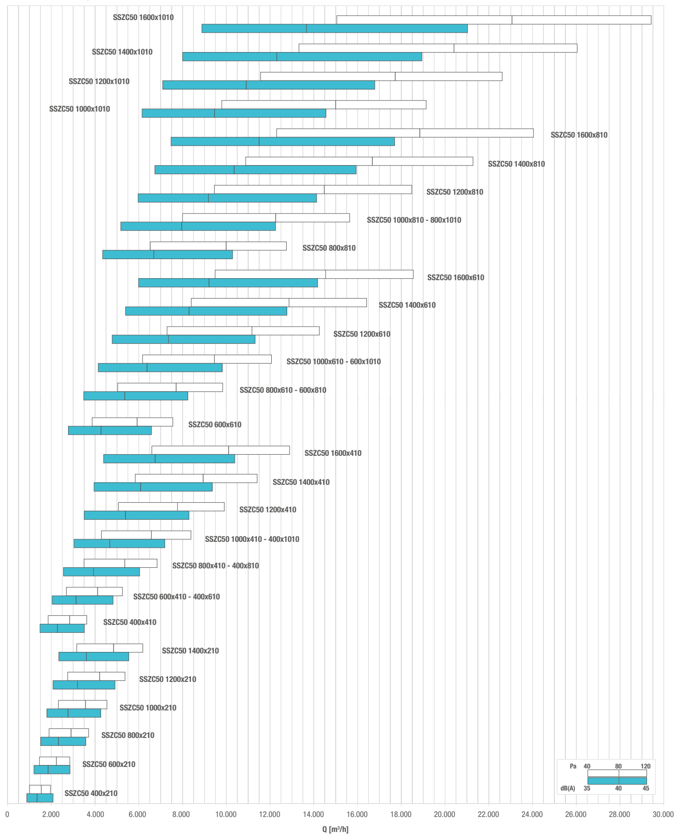
DIAGRAMĂ SELECȚIE RAPIDĂ - QUICK SELECTION DIAGRAM
