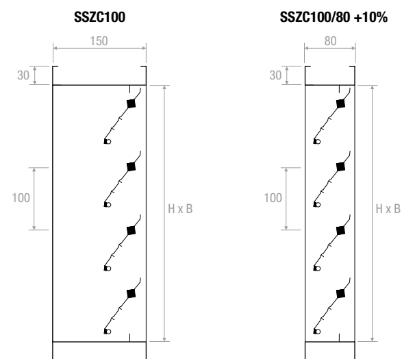
Lamele cu acționare conjugată +30% Blade with conjugate operation +30%
