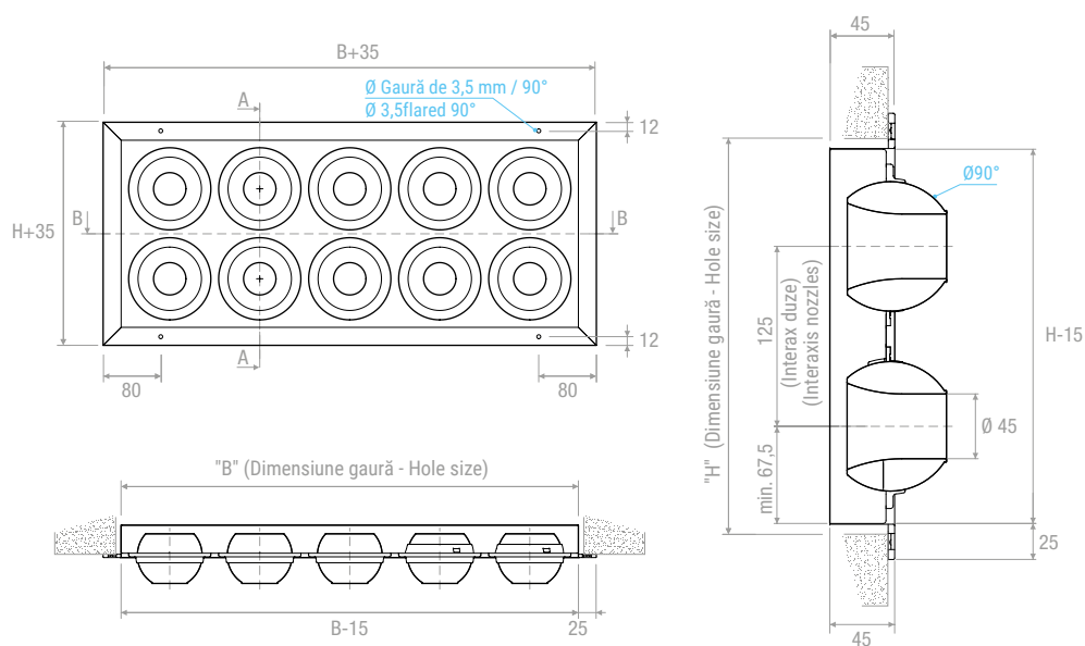
Secțiune - Section B-B
