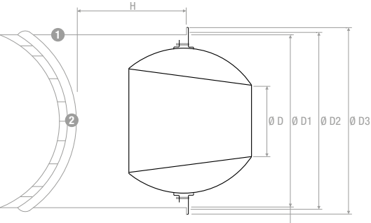
Montaggio su canale e su parete | Mounting on duct and at wall
