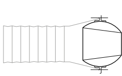
Montaggio con tubo flessibile Mounting by flexible duct
