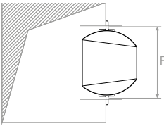
Montaggio su canale Mounting on the duct
