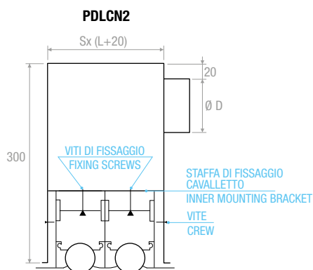
Fissaggio al plenum con staffe CVLCN cavalletti Fixing the plenum by inner mounting brackets CVLCN
