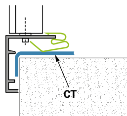
Fissaggio con plips
