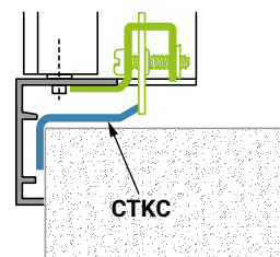
Fissaggio con morsetti KC
