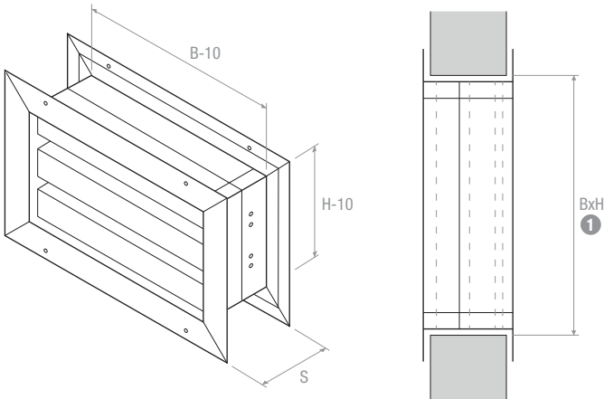
1 Dimensions du trou | Hole dimension
