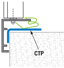
Fixation avec des clips Fixing with clips
