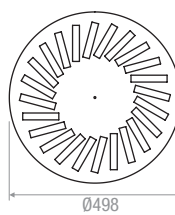
24 Fentes | Slots
