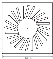
24 Fentes | Slots
