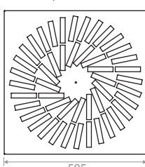
48 Fentes | Slots
