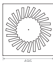
24 Fentes | Slots
