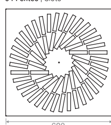
54 Fentes | Slots
