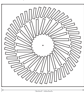
72 Fentes | Slots
