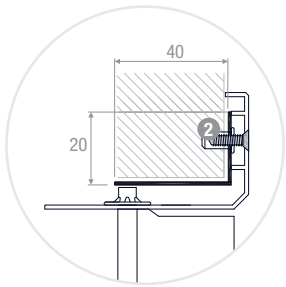
CTP BMAI Cadre avec crosses de fixation Frame with mounting brackets
