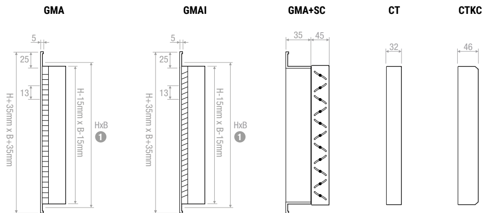
1 Dimensiones del orificio | Hole dimension
