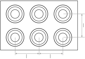
Montaje en batería Mounting on panel
