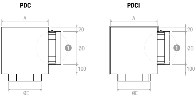
❶ Compuerta (bajo pedido) | Damper (on request) Plenum aislado externamente 6 mm de espesor Plenum externally insulated thickness 6 mm
