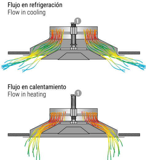
1 Elemento termostático | Thermostatic actuator
