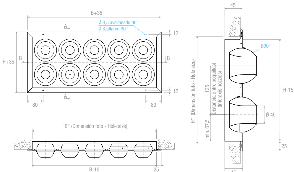
Sección - Section B-B
