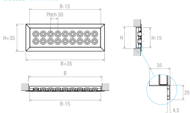
DIBUJOS - DRAWINGS
