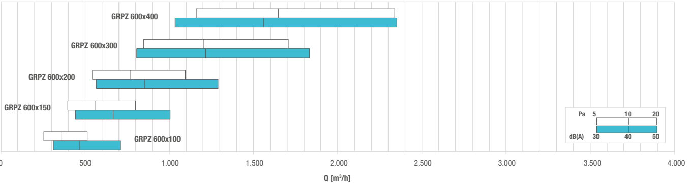
DIAGRAMA SELECCIÓN RÁPIDA - QUICK SELECTION DIAGRAM
