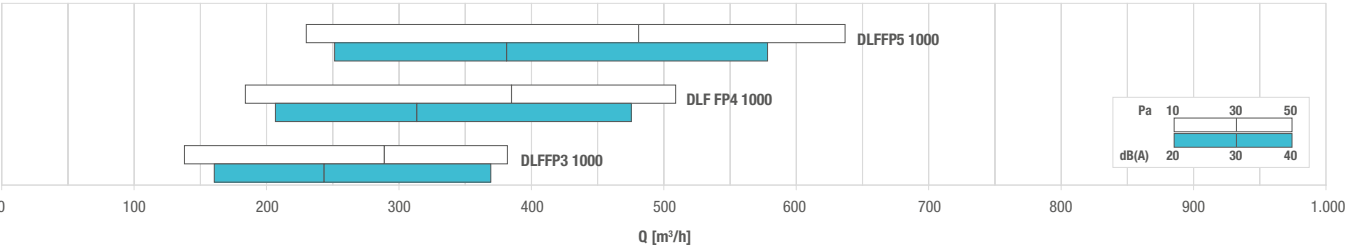
DIAGRAMA SELECCIÓN RÁPIDA - QUICK SELECTION DIAGRAM
