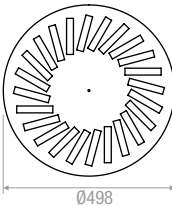
24 Feritoie | Slots
