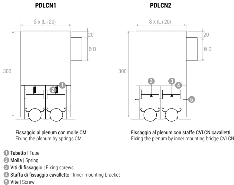
Posizionamento cavalletti CVLCN all'interno del plenum Positioning of bridge CVLCN inside plenum
