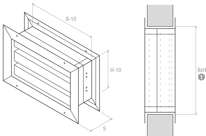
① Dimensioni foro | Hole dimension
