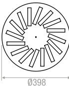
16 Feritoie | Slots
