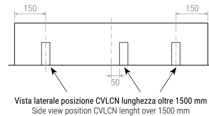
Centro plenum Plenum center
