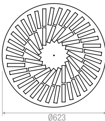
54 Feritoie | Slots
