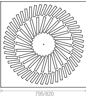
72 Feritoie | Slots
