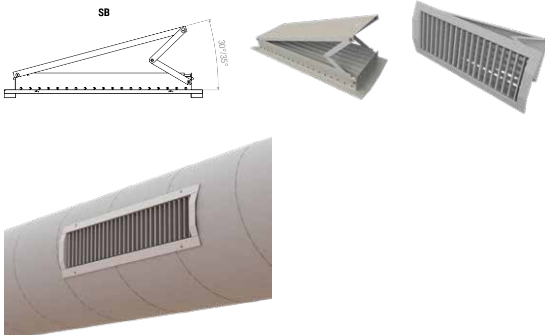
1 Sezione | Section
