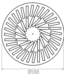
48 Feritoie | Slots
