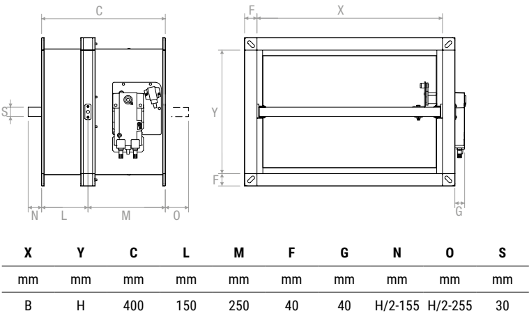
MDF30EUCEM Serranda tagliafuoco con predisposizione per servomotore Fire damper with predisposition for servomotor
