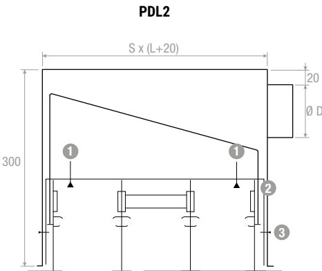
Fissaggio al plenum con staffe CVL cavalletti Fixing to the plenum by inner mounting bridge CVL
