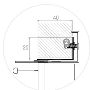
CTP BMI Telaio con zanche di fissaggio Frame with mounting brackets
