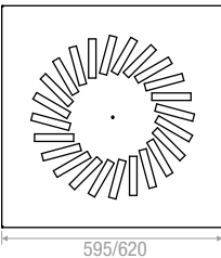
24 Feritoie | Slots
