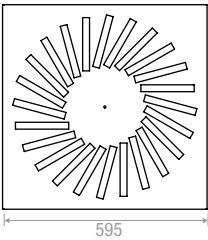
24 Feritoie | Slots
