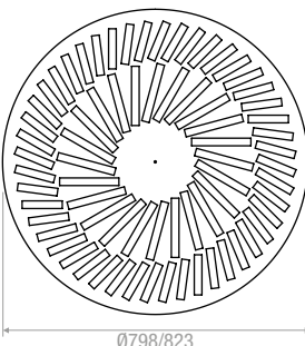
72 Feritoie | Slots
