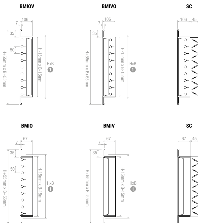
CTP BMI Telaio con zanche di fissaggio Frame with mounting brackets
