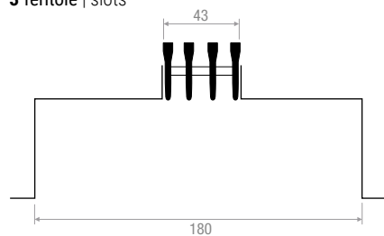
3 feritoie | slots
