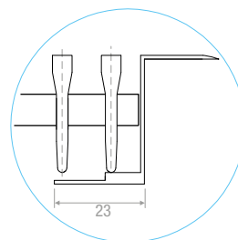
DETAIL LAMELLENAUFNABME AUF DEM RAHMEN PARTICULAR HOUSING BARS ON FRAME
