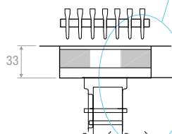
DETAIL KLAPPENAUFNABME AUF DEM RAHMEN PARTICULAR HOUSING DAMPER ON FRAME
