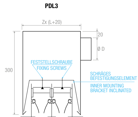
Befestigung am Anschlusskasten mit geneigten Montagestegen CVL Fixing to the plenum by inner mounting brackets inclined CVL
