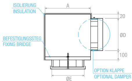
PLENUM PDCQI
