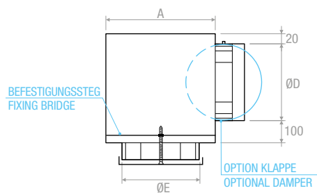
ANSCHLUSSKASTEN PDCQ
