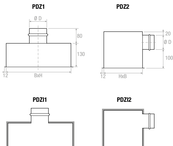
Anschlusskasten mit 6 mm Außenisolierung Plenum externally insulated thickness 6 mm
