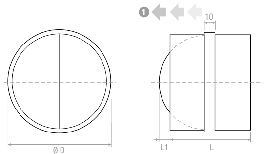
1 Luftstrom | Air flow
