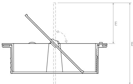
Abschnitt | Section A-A
